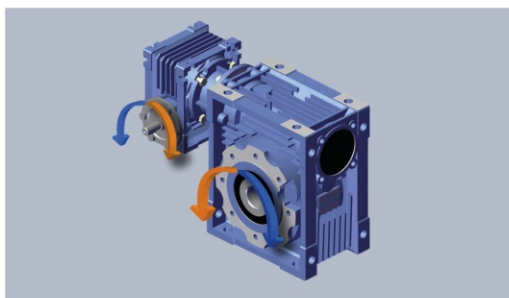
EINBAULAGE BS1
