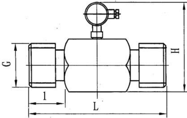
图 2 螺纹连接结构
