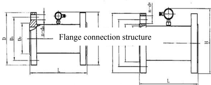
图3 法兰连接结构
