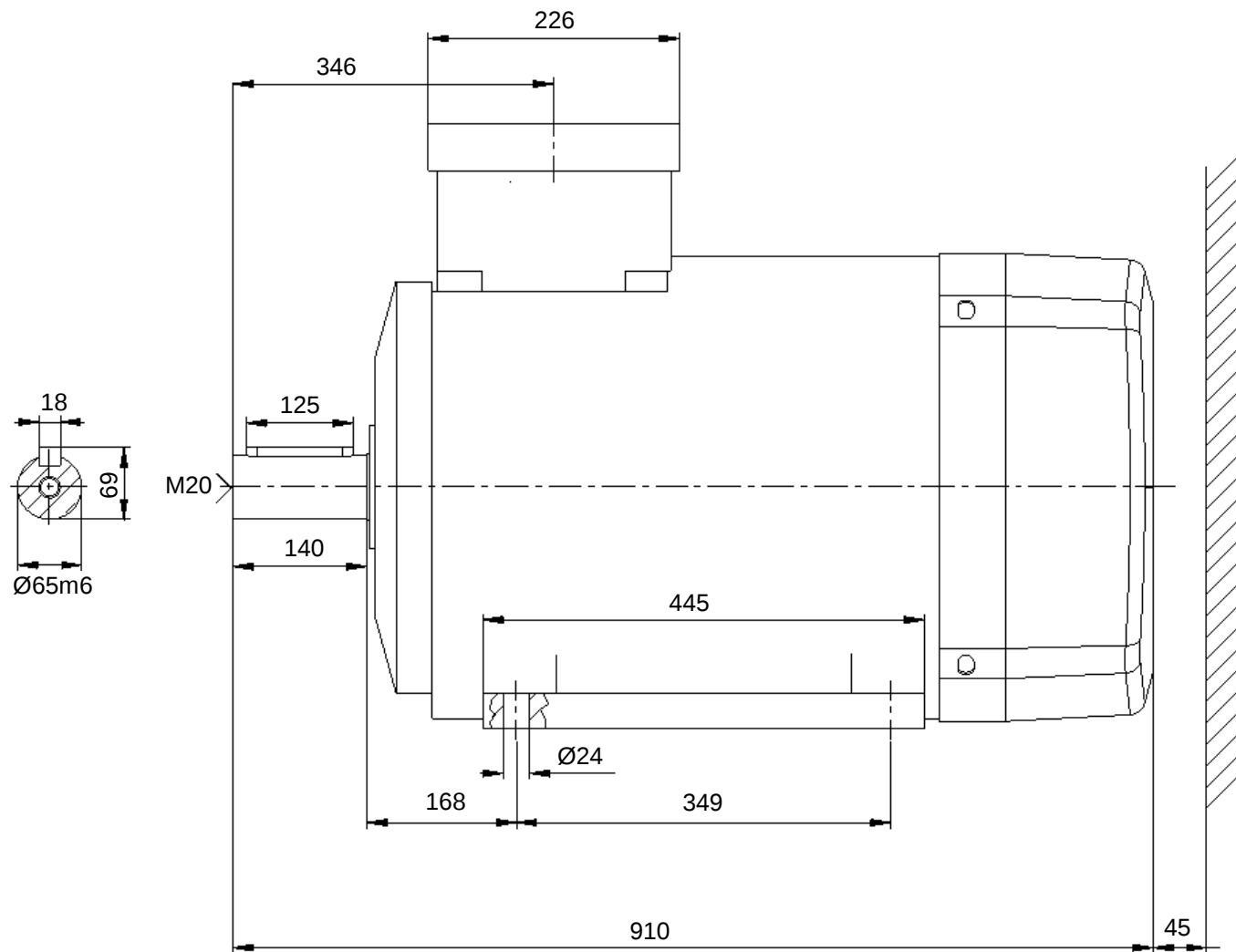
Maßblatt - #713348 - KDG2C 250 M 4 KT NV VL IE3 in Angebot An181147 Position 1 Kabelverschraubung: 2x M63x1,5
