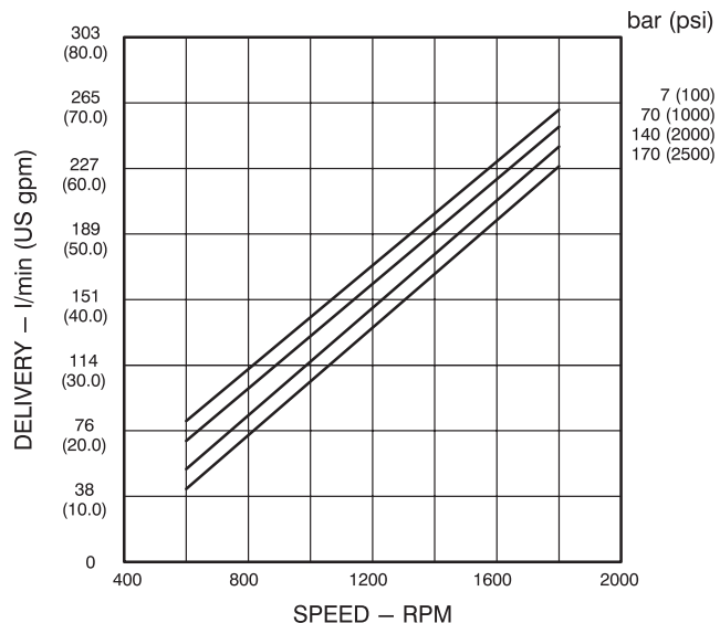
Code 45 Displacement
